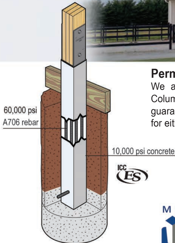
Precast Perma-Column®
